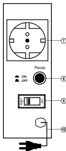
Рис. 3. Боковая стенка* AVR SLIM-500 LCD, AVR SLIM-1000 LCD
