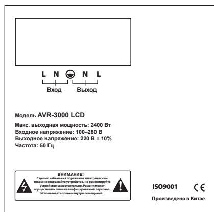
AVR-3000 LCD**
