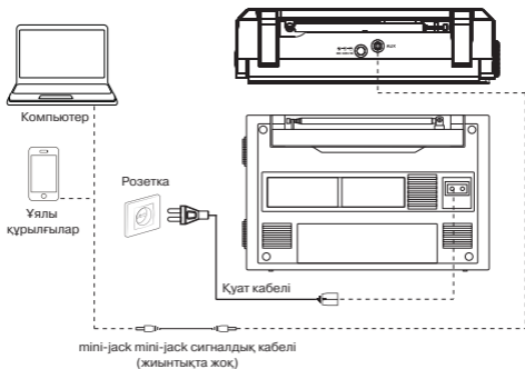
3-сурет. Қосылу схемасы
