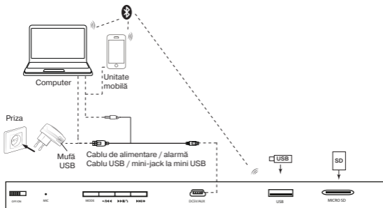
Imag. 2. Schema conectării
