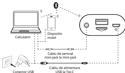
Fig. 2. Schema de conexiuni
