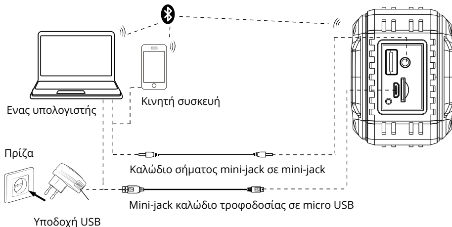
Εικ. 2. Σχέδιο σύνδεσης
