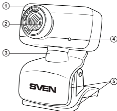
Мал. 1. Будова веб-камери
