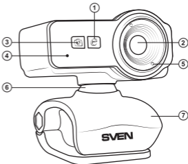
1-сурет. Веб-камераның құрылысы
