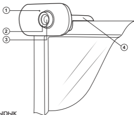
1-сурет. Веб-камераның құрылысы
