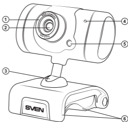
1-сурет. Веб-камераның құрылысы
