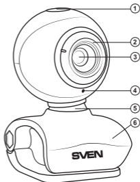
Рис. 1. Устройство веб-камеры
