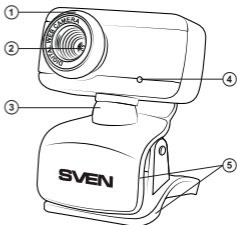
1-сурет. Веб-камераның құрылысы
