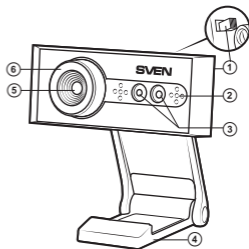
Рис. 1. Устройство веб-камеры
