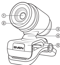
Рис. 1. Устройство веб-камеры
