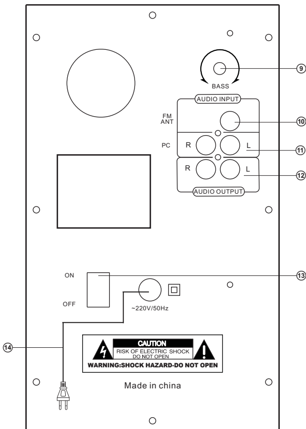
2-сурет. Сабвуфердің артқы панелі
