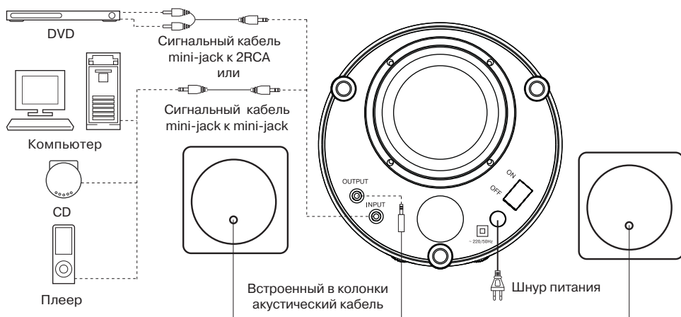
Рис. 3. Схема подключения
