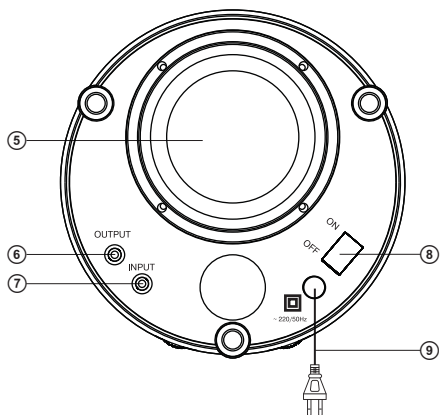
Рис. 2. Нижняя панель сабвуфера
