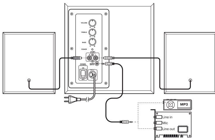
Рис. 2. Схема подключения
