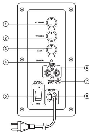
Рис. 1. Панель управления
