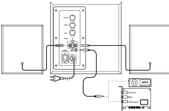
Мал. 2. Схема підключення
