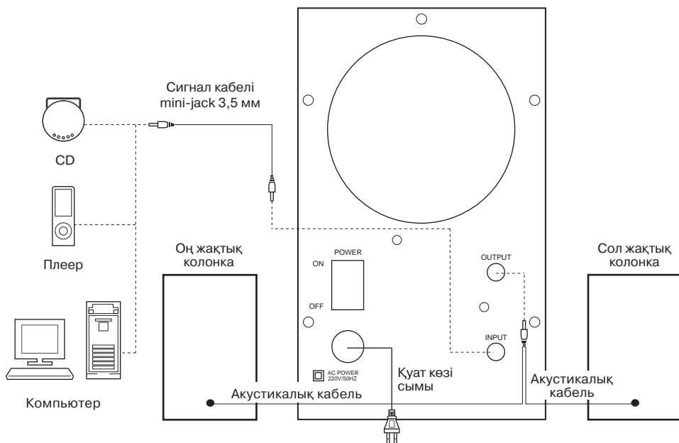
3-сурет. Қосылу схемасы
