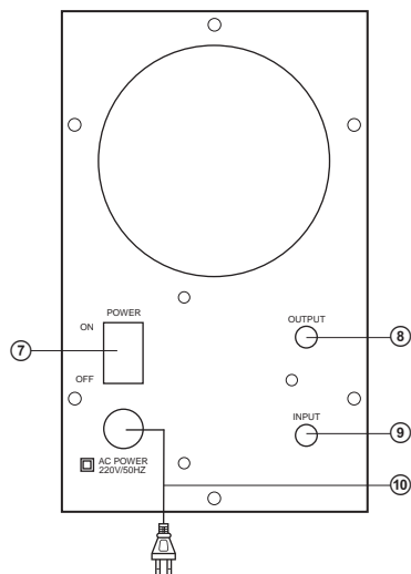
2-сурет. Сабвуфердің артқы панелі
