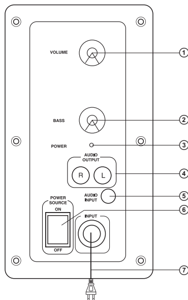
Imag. 1. Panoul din spate al subwooferului
