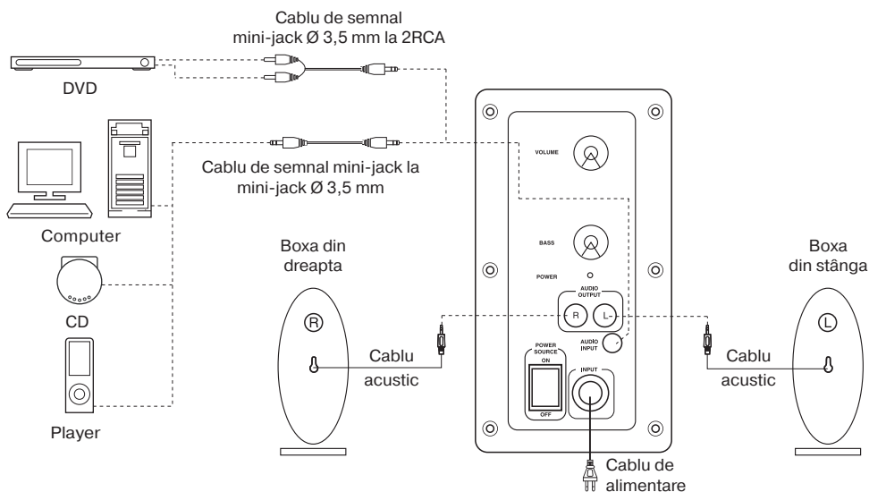
Imag. 2. Schema conectării
