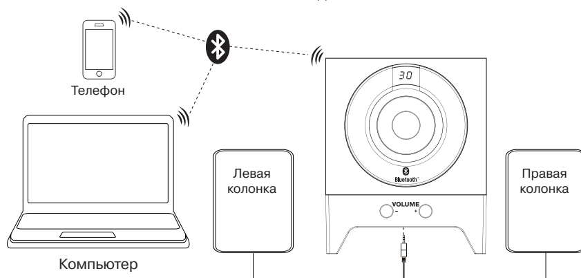
Рис. 5. Схема с подключением Bluetooth-модуля
