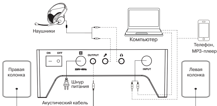
Рис. 4. Схема подключения
