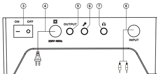
Рис. 2. Задняя панель сабвуфера
