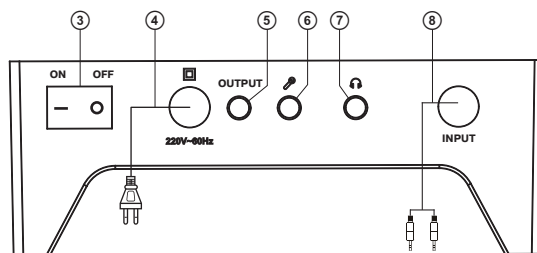
Мал. 2. Задня панель сабвуфера
