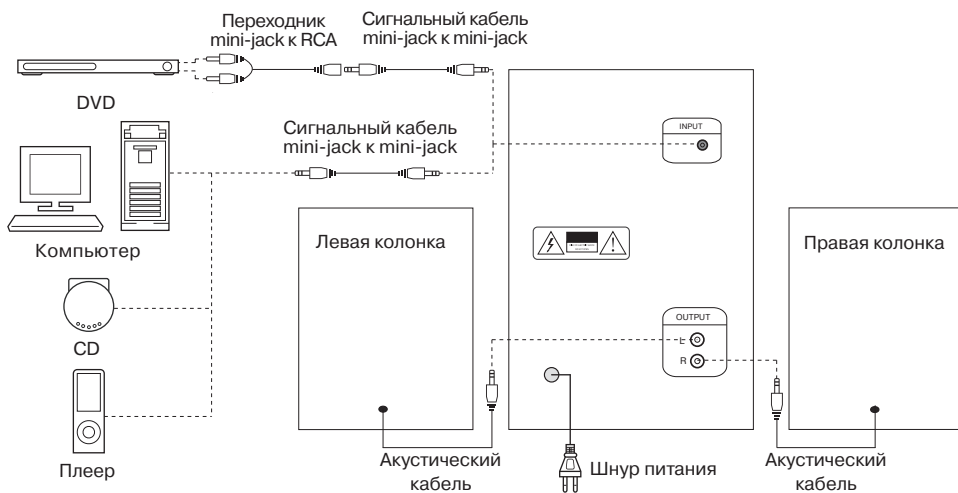
Рис. 3. Схема подключения
