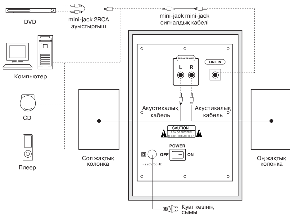
3-сурет. Қосылу схемасы
