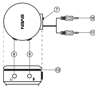
2-сурет. ДБ пульты
