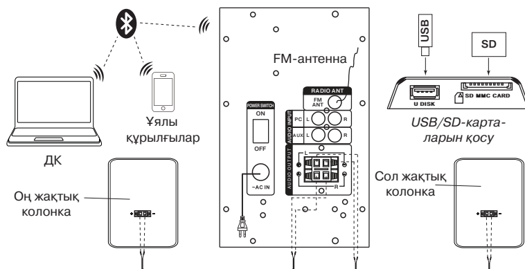
6-сурет. Қосылу схемасы Bluetooth-модулі
