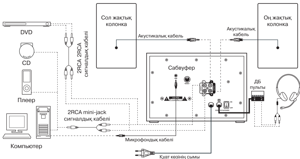
2-сурет. Қосылу схемасы
