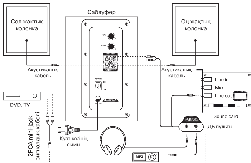
3-сурет. Қосылу схемасы
