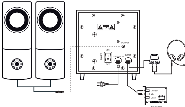
2-сурет. Қосу схемасы
