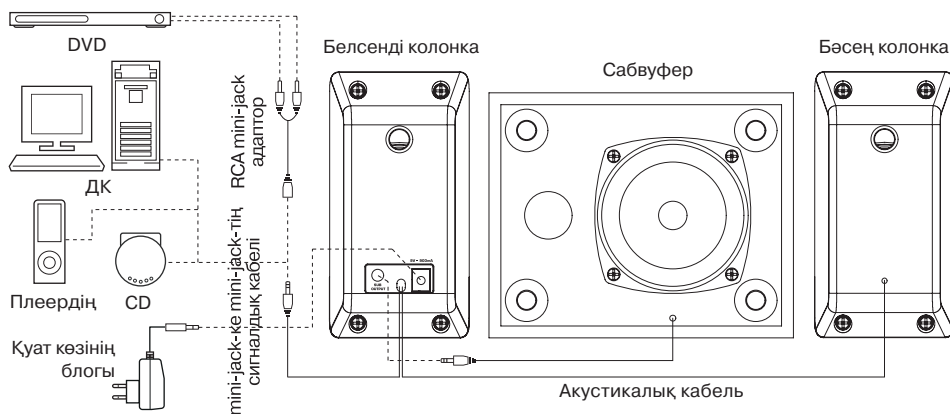
2-сурет. Қосылу схемасы
