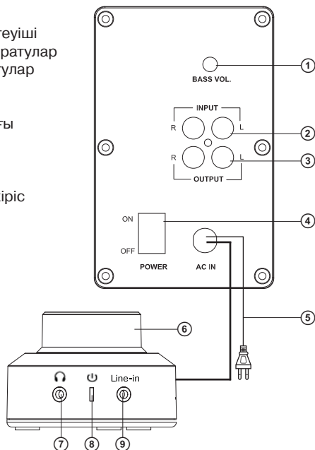
1-сурет. Сабвуфердің артқы панелі
