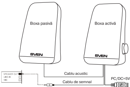
Imag. 2. Schema conectării
