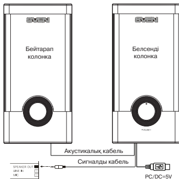
2-сурет. Қосу схемасы
