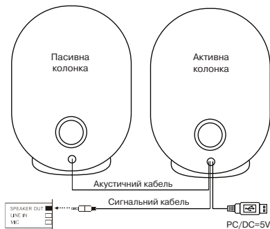
Мал. 2. Схема підключення
