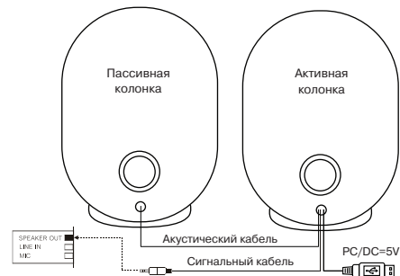
Рис. 2. Схема подключения
