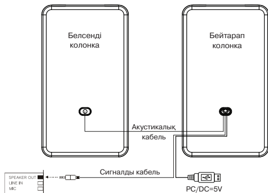
2-сурет. Қосу схемасы
