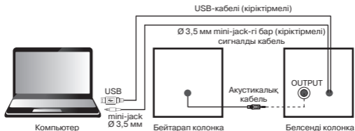
2-сурет. Қосу схемасы
