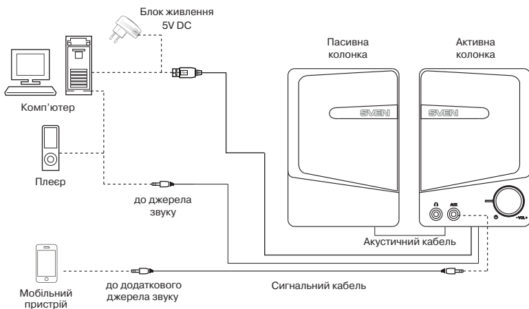
Мал. 2. Схема підключення
