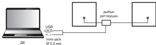
Қосу схемасы
