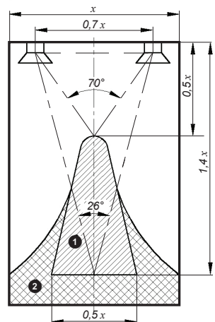
Мал. 1. Схема розташування АС
