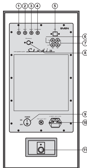
Рис. 3. Задняя панель
