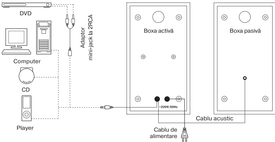
Imag. 2. Schema conectării
