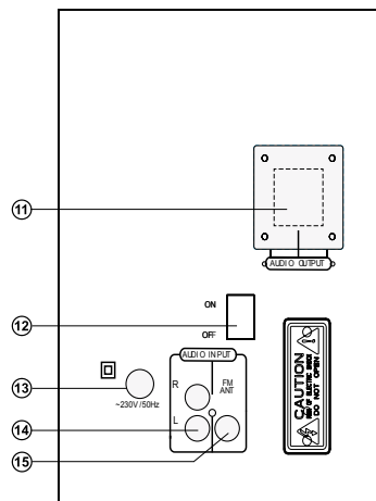
Мал. 2. Задня панель активної колонки
