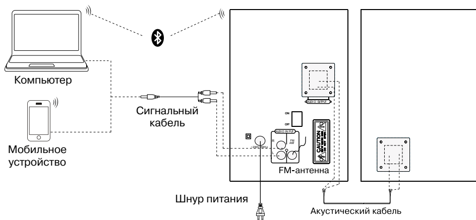
Рис. 4. Схема подключения источников аудиосигнала
