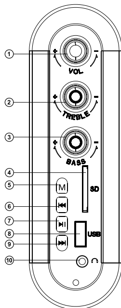
Рис. 1. Панель управления
