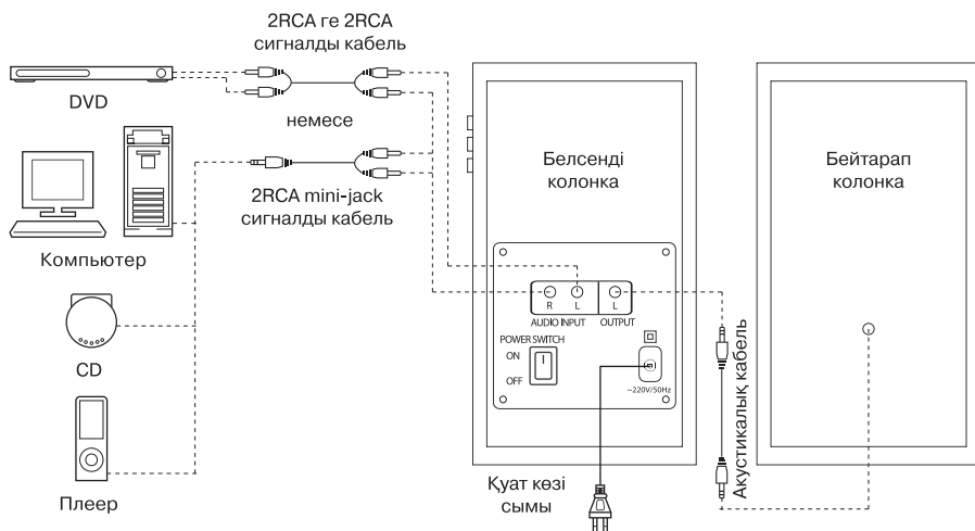
2-сурет. Қосу схемасы
