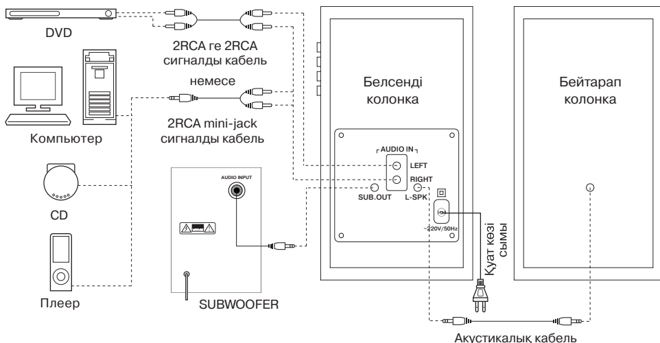
2-сурет. Қосу схемасы
