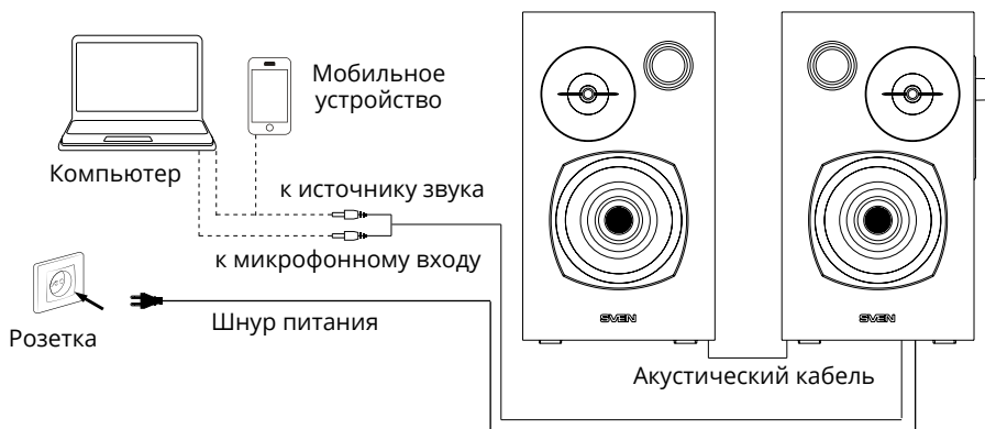
Рис. 2. Схема подключения
