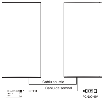
Imag. 2. Schema conectării
