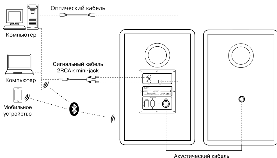
Рис. 4. Схема подключения
