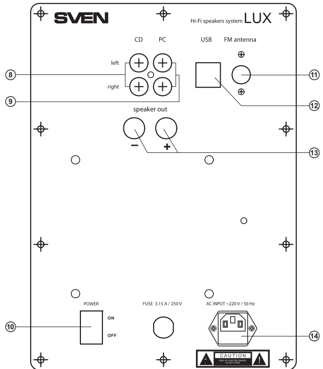
Мал. 3. Задня панель активної колонки
