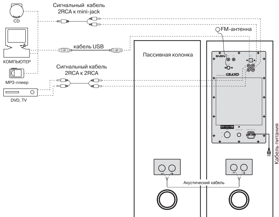
Рис. 5. Схема подключения
