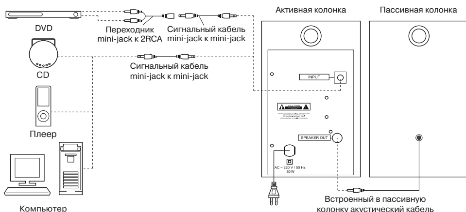
Рис. 3. Схема подключения
