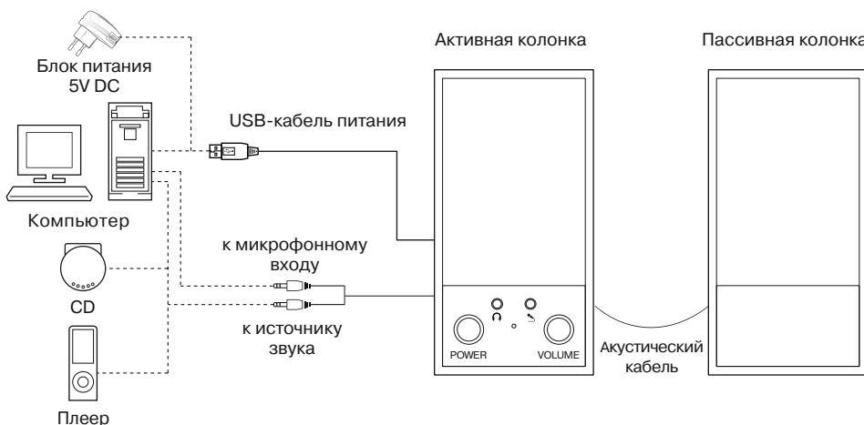
Рис. 2. Схема подключения
