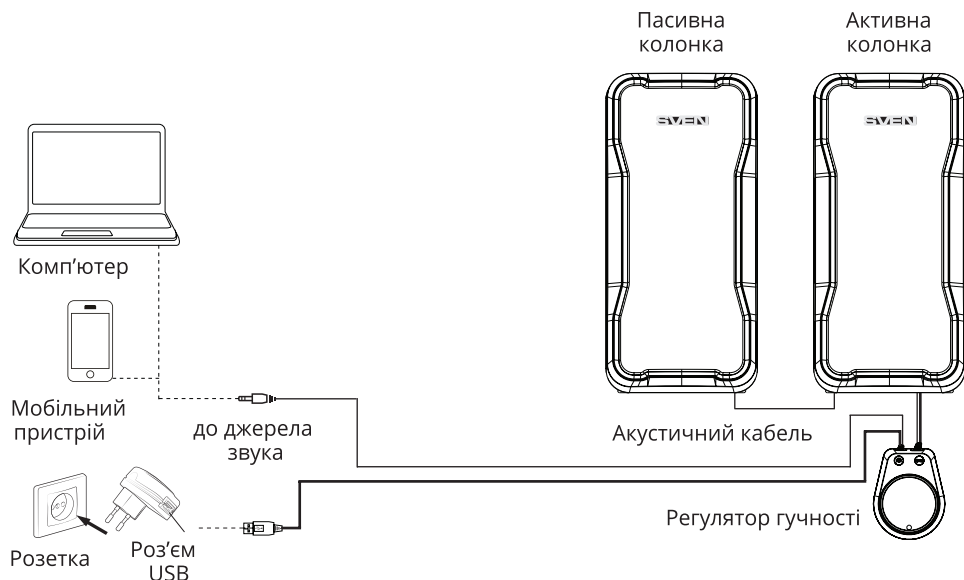
Мал. 2. Схема підключення
